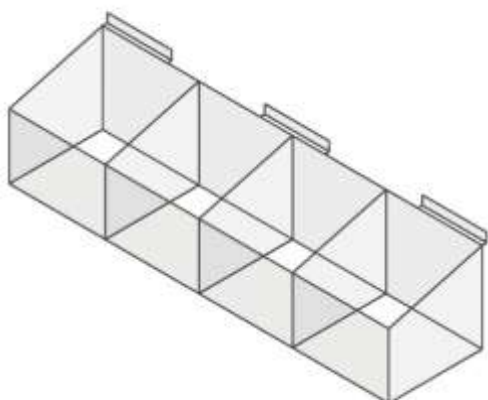
Contenitore 4 tasche P 20 x L 59 x H 15
